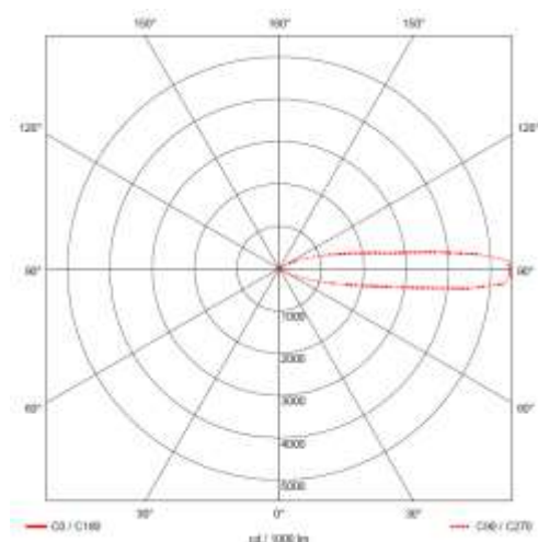
Illustrazione 5: Caratteristica di emittenza luce piena
